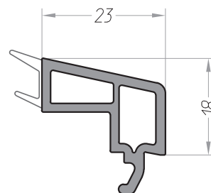
Штапик 23 арт. 10104023 - черное уплотнение арт. 10204023 - серое уплотнение арт. 10204023.5 - т-серое уплотнение
