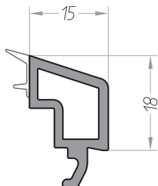
Штапик 15 AERO арт. 10004015 - черное уплотнение
