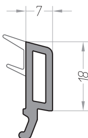
Штапик 7 арт. 10404007 - черное уплотнение арт. 10204007 - серое уплотнение арт. 10204007.5 - т-серое уплотнение
