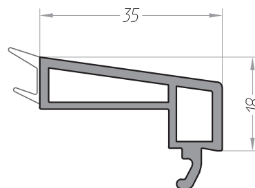
Штапик 35 арт. 10104035 - черное уплотнение арт. 10204035 - серое уплотнение арт. 10204035.5 - т-серое уплотнение
