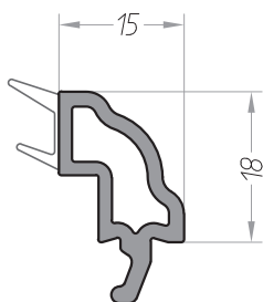
Штапик 15 фигурный арт. 10904015 - черное уплотнение арт. 10904015.3 - серое уплотнение арт. 10904015.5 - т-серое уплотнение
