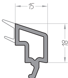
Штапик 15 арт. 10404015 - черное уплотнение арт. 10204015 - серое уплотнение арт. 10204015.5 - т-серое уплотнение
