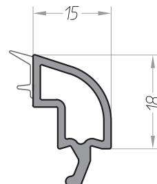
Штапик 15 круглый арт. 10604015 - черное уплотнение
