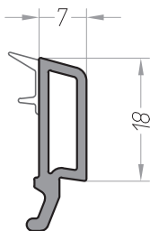
Штапик 7 AERO арт. 10004007 - черное уплотнение
