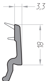
Штапик 3 GLIDE арт. 10804003 - черное уплотнение арт. 10804003.3 - серое уплотнение
