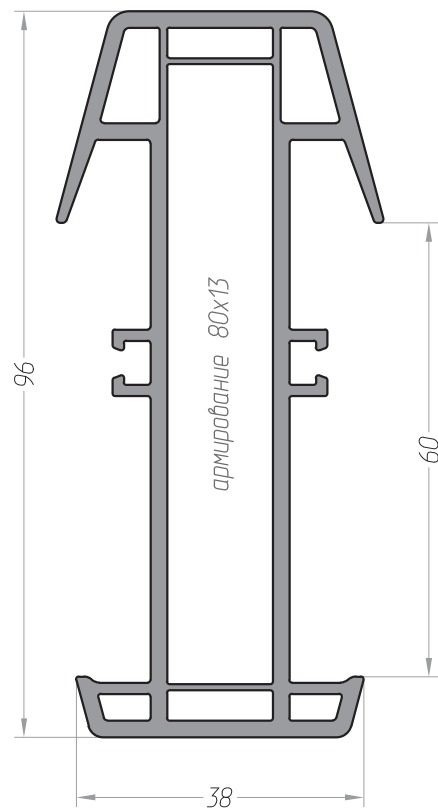
Профиль соединительный 38/60 арт. 10105038
